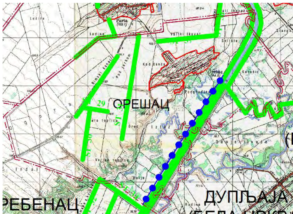
Слика 9: Могући распоред пољозаштитних шумских појасева на КО Орешац
